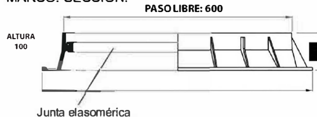
MARCO. SECCIÓN.
